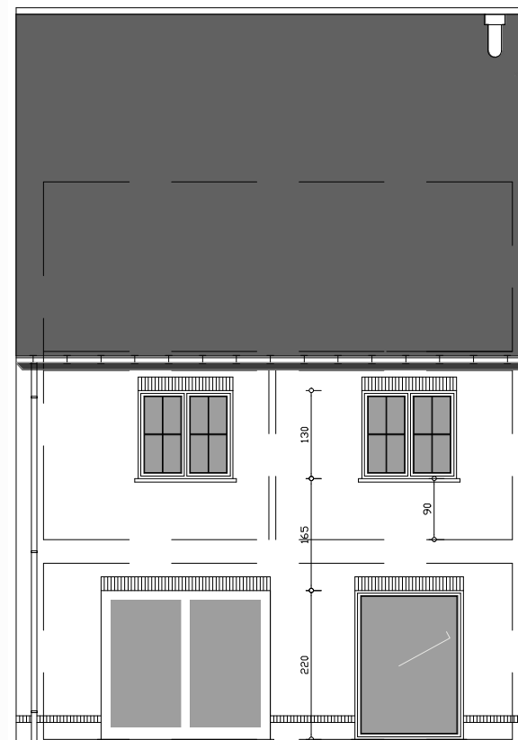
voorgevel
